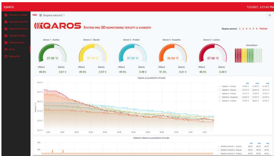
Konfigurace sady a vizualizace měřených údajů
